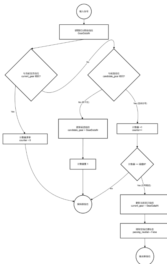
图 4.3 挡传滤波算法流程图
